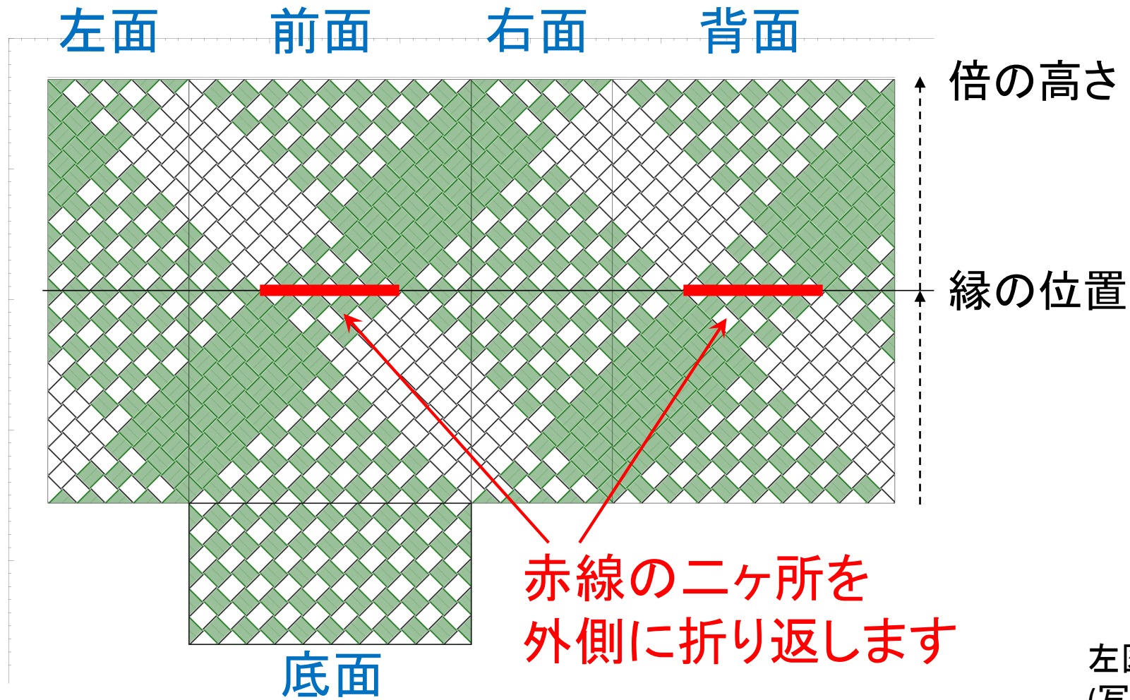
外側から見た側面の展開図(高さの2倍分)
